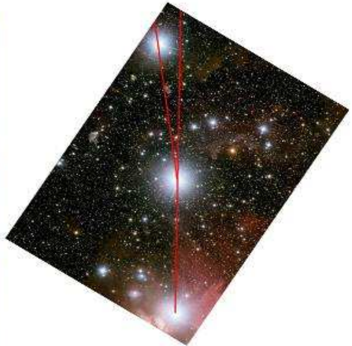
Constelación de Orion
